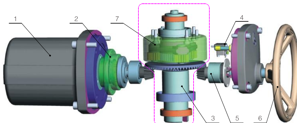
电动执行器主要结构
