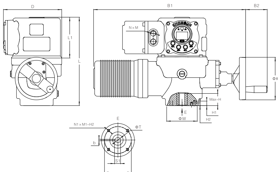
CSR - G03 系列电动执行器 机构主要尺寸及法兰连接尺寸
