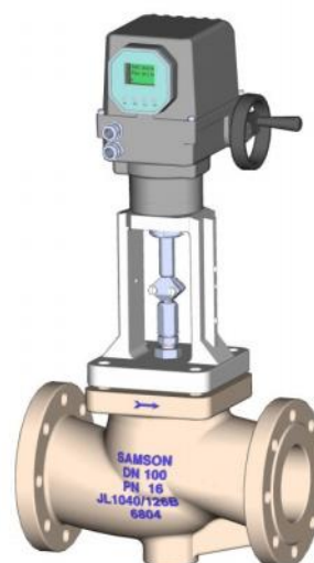
CSL-G02系列直行程电动执行器 (装配于SAMSON3241- DN100型单座调节阀)
