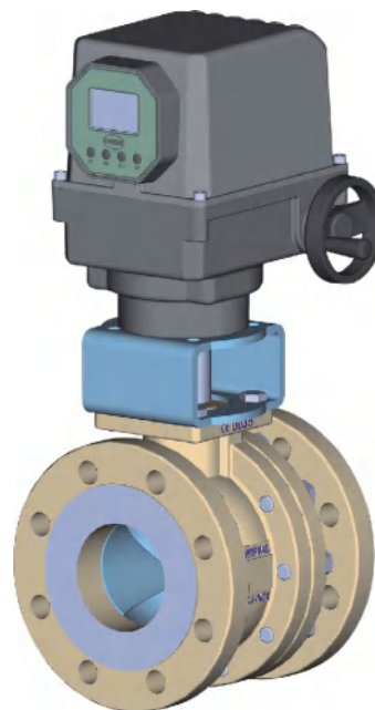
CSR-G02系列 角行程电动执行器 (装配于CHEMSUN V型调节球阀)
