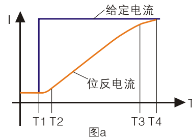
图a: 给定电流与位置反馈电流变化关系图
