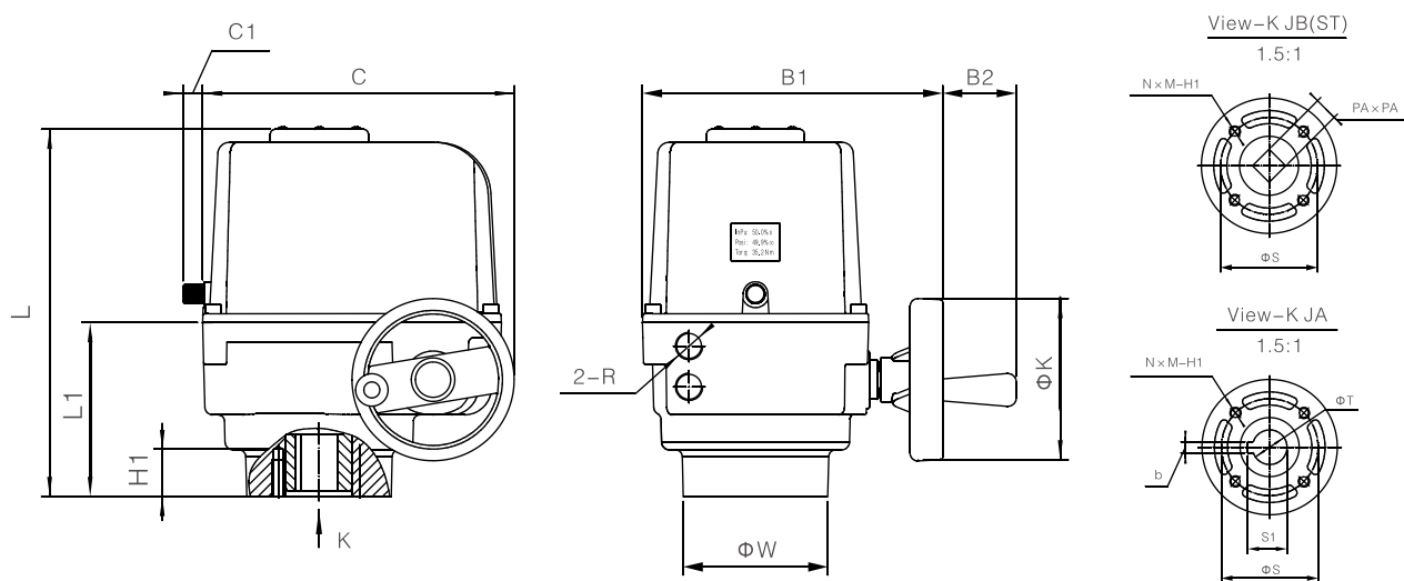
CSR/L - G02系列电动执行机构主要尺寸及法兰连接尺寸
