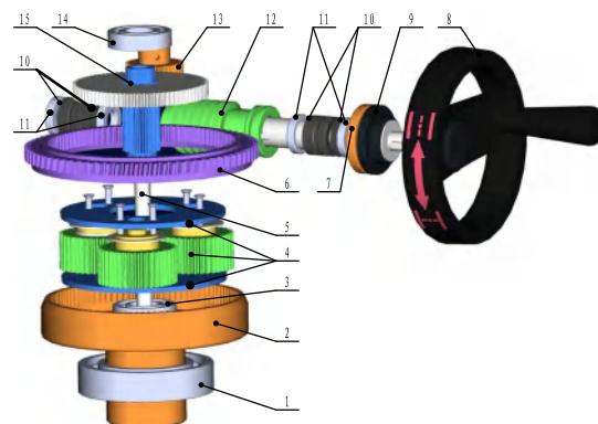
机械结构及齿轮传动系
