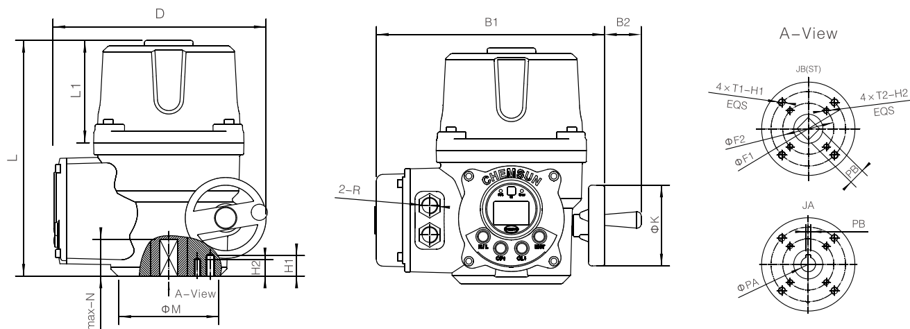
CSR/L-G01系列电动执行机构主要尺寸及法兰连接尺寸
