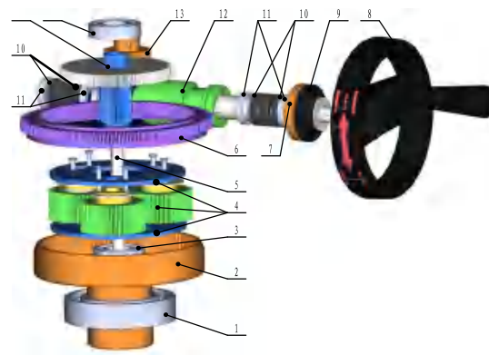
机械结构及齿轮传动系
